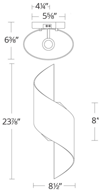
WS-W34524
